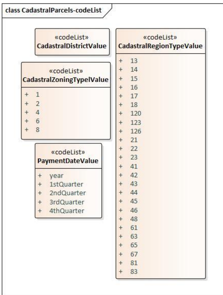
С.4-р зураг - UML диаграмм: Кадастрын нэгж талбар багцын кодын жагсаалт
