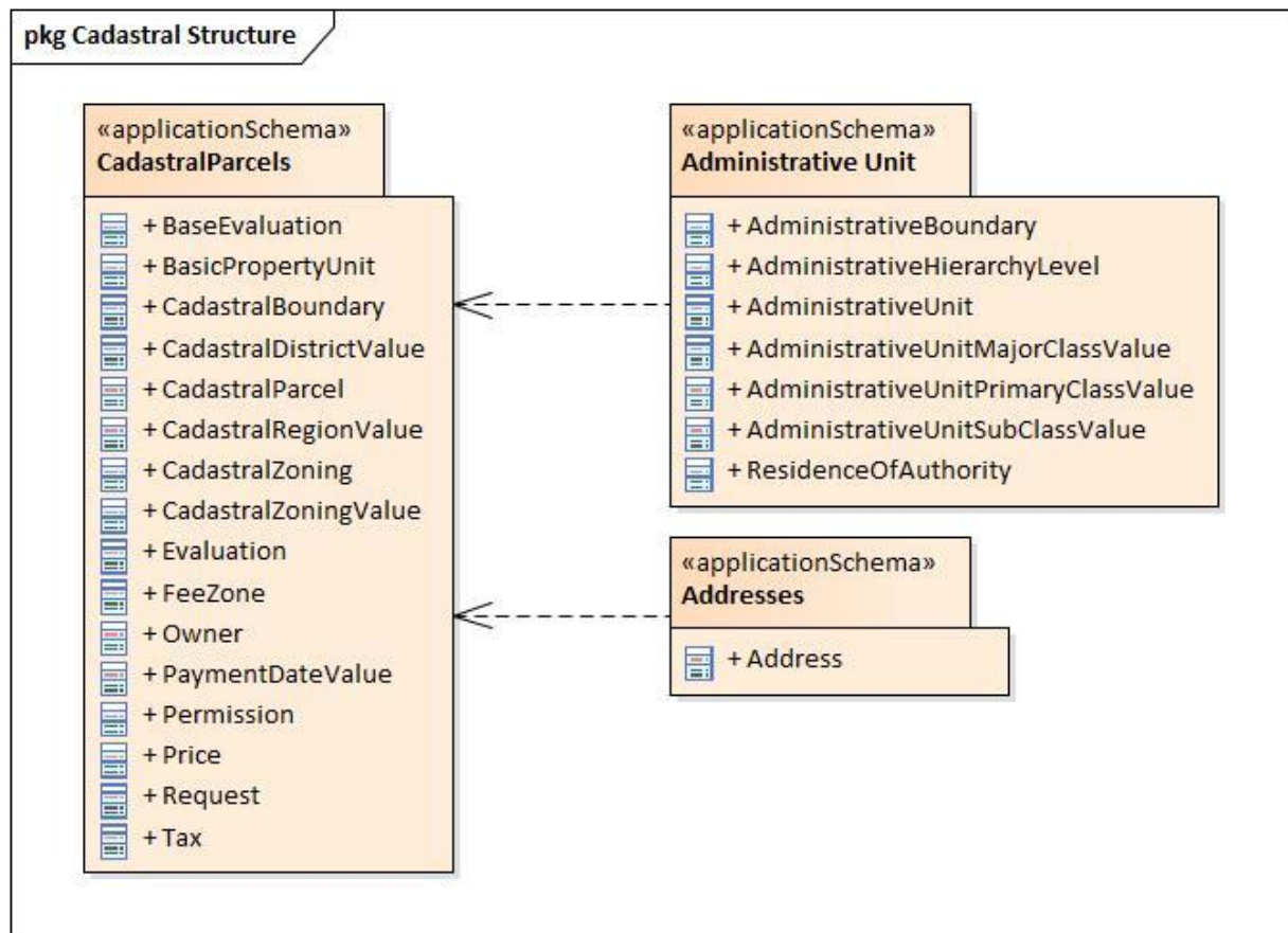
С.1-р зураг - UML диаграмм: Кадастрын нэгж талбар багцын хэрэглээний схемийн тойм
